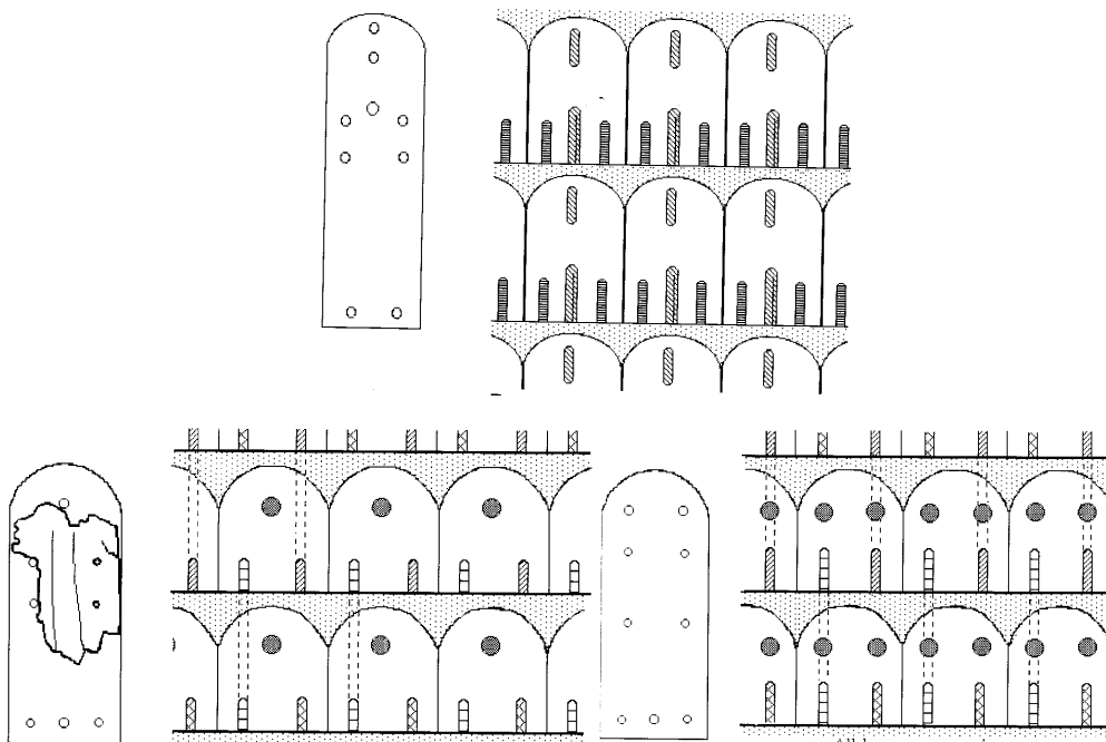
Εικόνα 4. Σχηματική αναπαράσταση της εξέλιξης της κατασκευής του κλιβανίου με τη χρήση δερμάτινου υποστρώματος. Με τις πλάκες ραμμένες στο υπόστρωμα (πάνω), ενωμένες στο δέρμα με μονό πριτσίνι (αριστερά) ή με διπλό (δεξιά).
