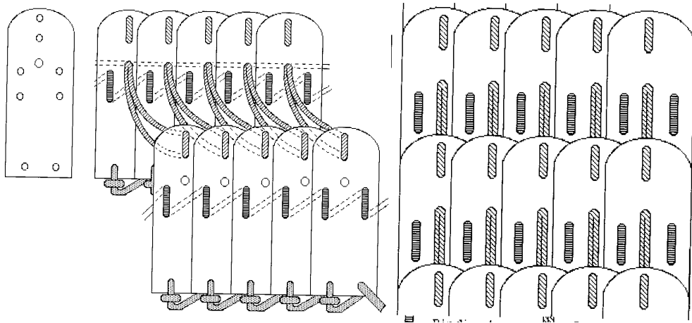
Εικόνα 3. Σχηματική αναπαράσταση του τρόπου δεσίματος των πλακών του κλιβανίου.
