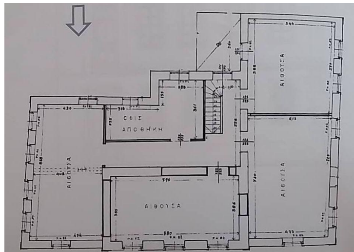
κάτοψη ισογείου
