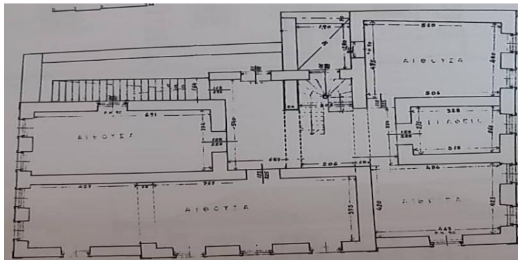
κάτοψη πρώτου ορόφου
