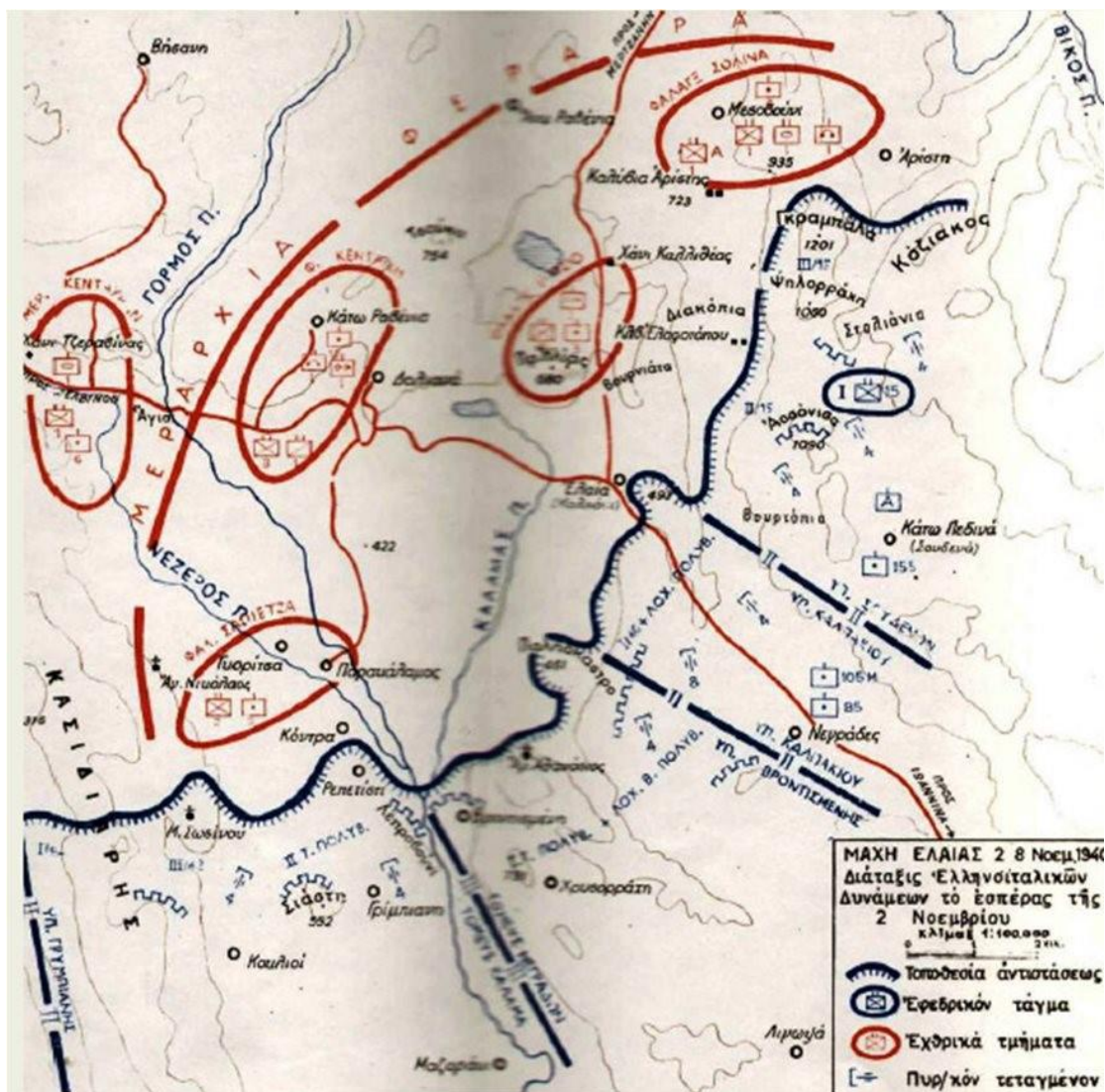
Σχεδιάγραμμα της μάχης Ελαία-Καλαμά. ΓΕΣ/ΔΙΣ, Ο Ελληνικός Στρατός κατά τον Δεύτερον Παγκόσμιον Πόλεμον. Ο Ελληνοϊταλικός Πόλεμος 1940-41, Η Ιταλική Εισβολή, Αθήνα 1960, σχεδιάγραμμα 4.
